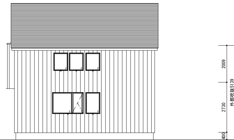
東側立面図
