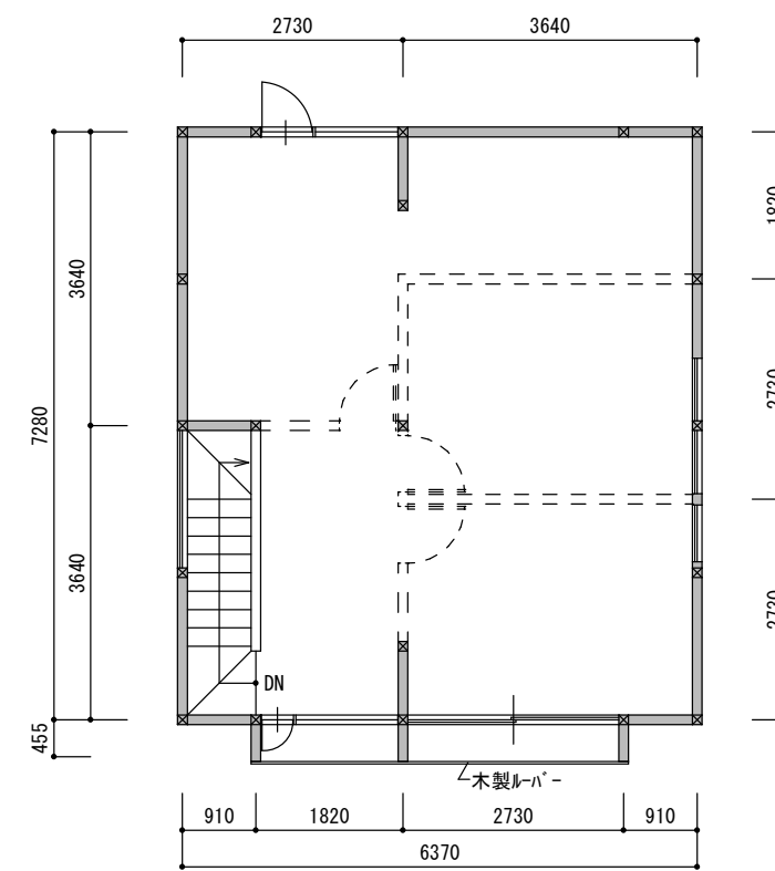
2階平面図
