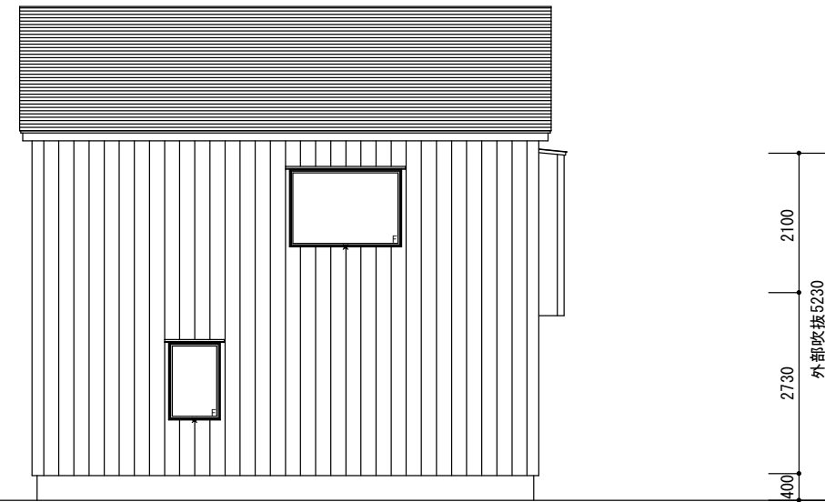
西側立面図
