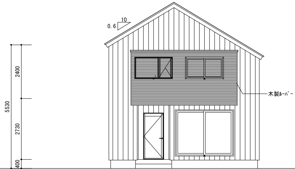
南側立面図
